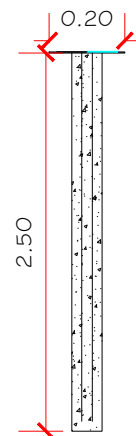
CORTE - ESTACA
