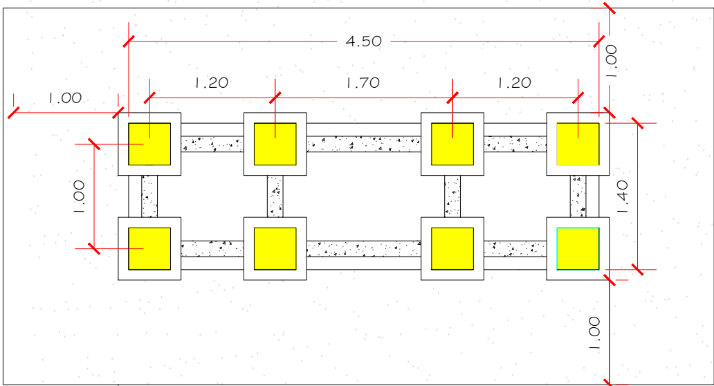
ESTACAS 0,20x0,20
